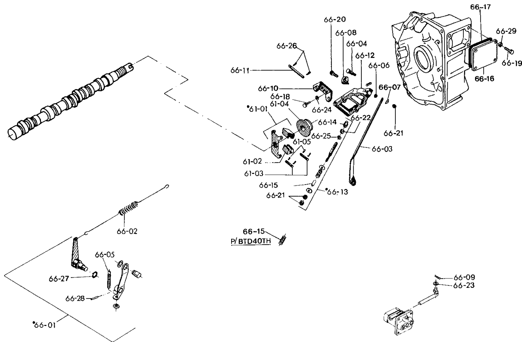
SISTEMA DE GOVERNADOR - SISTEMA REGULADOR
